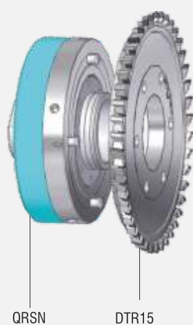
Primjer montaže na brzoizmjenjivu steznu čahuru
