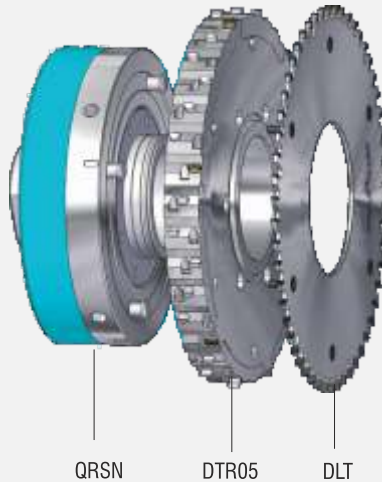
Primjer montaže na brzoizmjenjivu steznu čahuru
