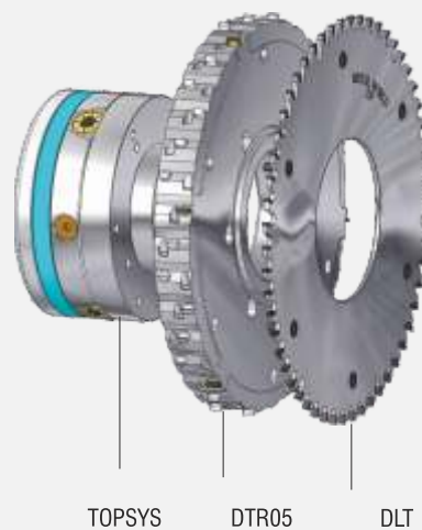
Primjer montaže na „Top System“ steznu čahuru
