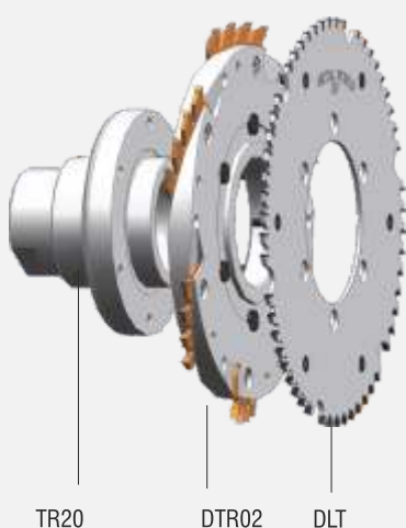
Primjer montaže na standardnu steznu čahuru
