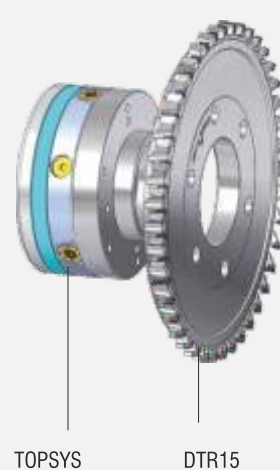
Primjer montaže na „Top System“ steznu čahuru
