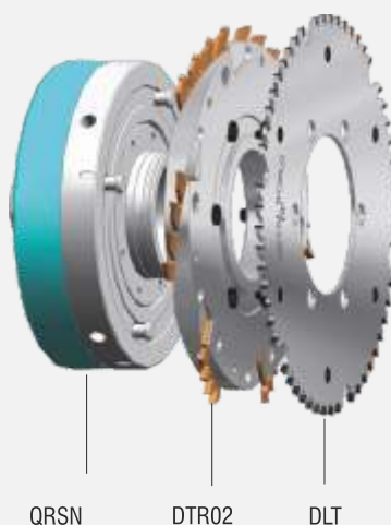
Primjer montaže na brzoizmjenjivu steznu čahuru
